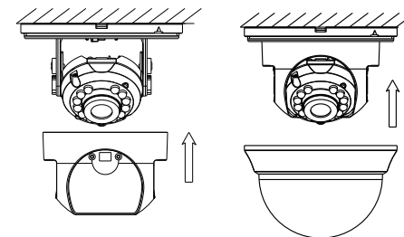
Рисунок 2-12 Завершение установки
