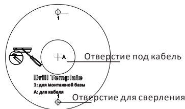
Рисунок 2-9 Шаблон крепления
