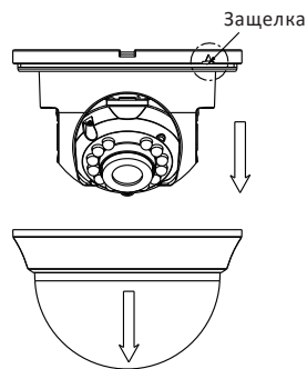
Рисунок 2-8 Снятие купола
