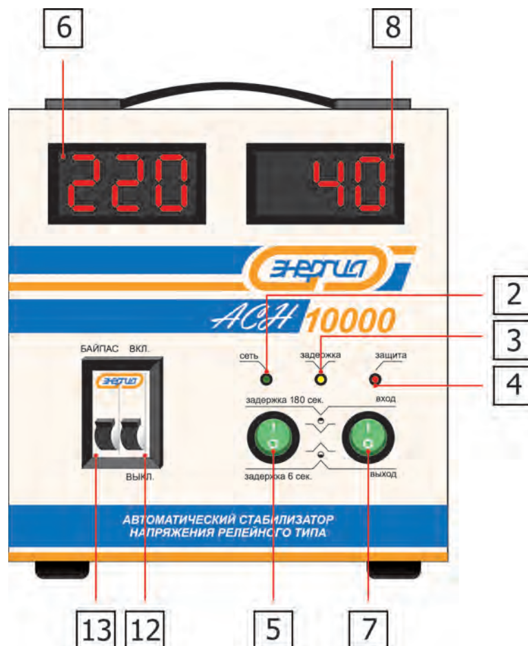
Лицевая панель
